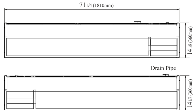
SAKURA-70R / SAKURA-70L TOP VIEW
